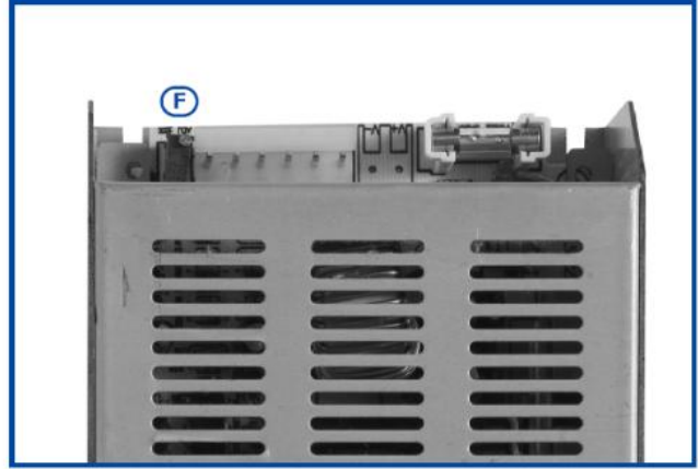
5A-es kapcsolóüzemű tápegység (SmartLiving 10100L)
