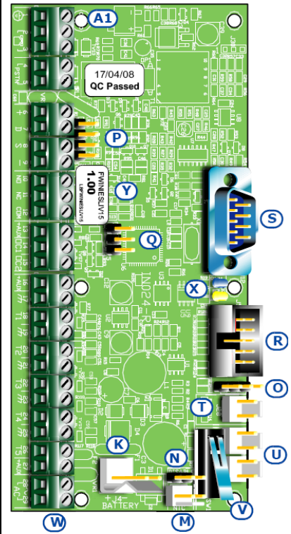
A SmartLiving515 központ alaplappja
