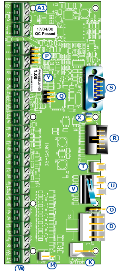
A SmartLiving 1050 / 1050L és 10100L központ alaplappja
